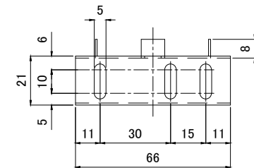
取付金具
