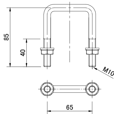
コ型ボルト(オプション)
